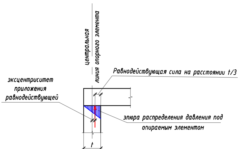
Схема передачи вертикального усилия на опорный элемент при прямом опирании без закладных деталей
