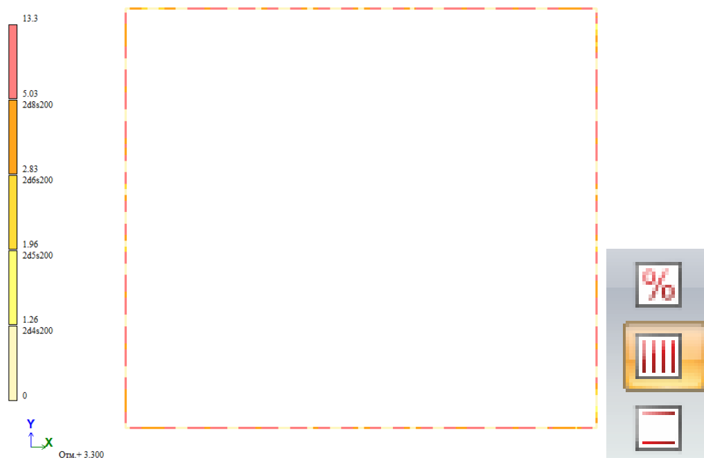
Рисунок. Требуемое поперечное армирование балок. Вертикальное направление.
