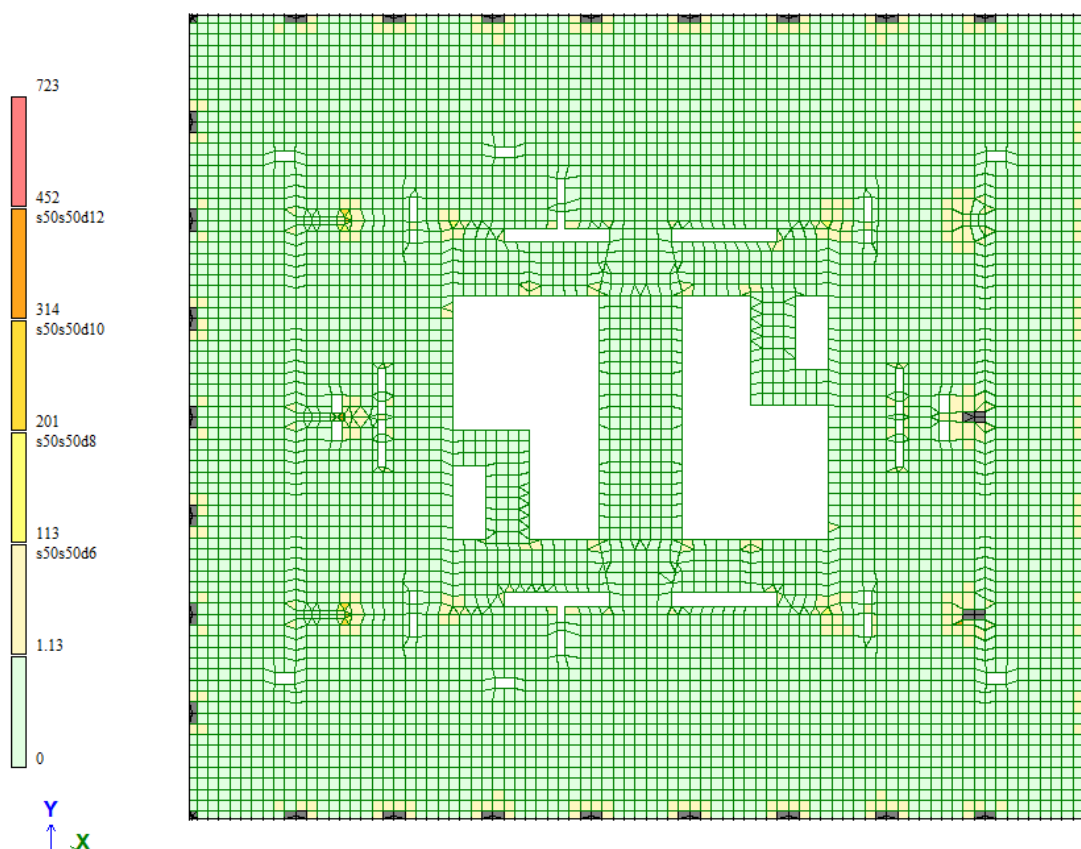
Рисунок. Требуемое поперечное армирование плит на 1м².
